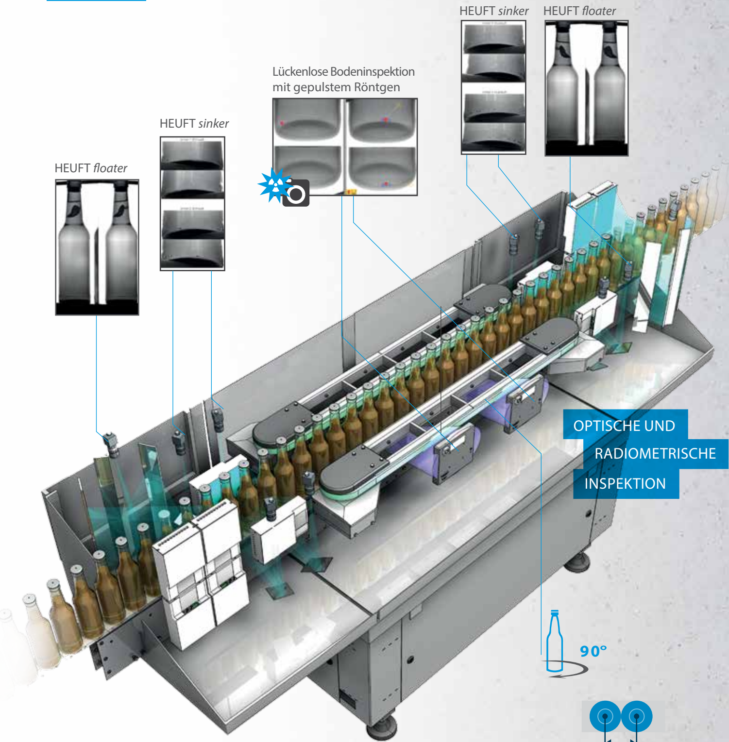
Sichere Rundum-Inspektion auch bei lückenlosem Flaschenfluss
